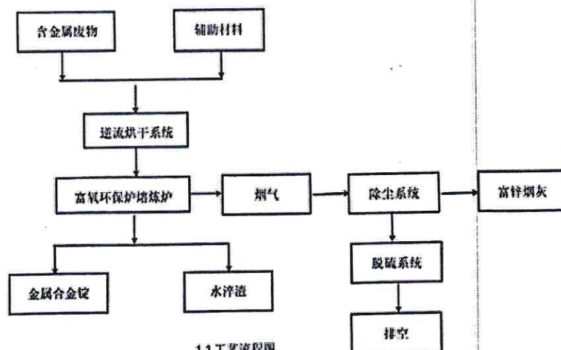
1.1 工艺流程图
