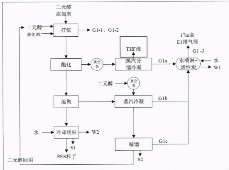
图 2: PES 工艺流程图。
