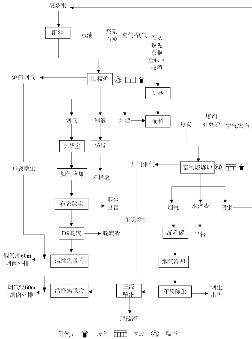
富氧熔炼炉工艺流程见图
